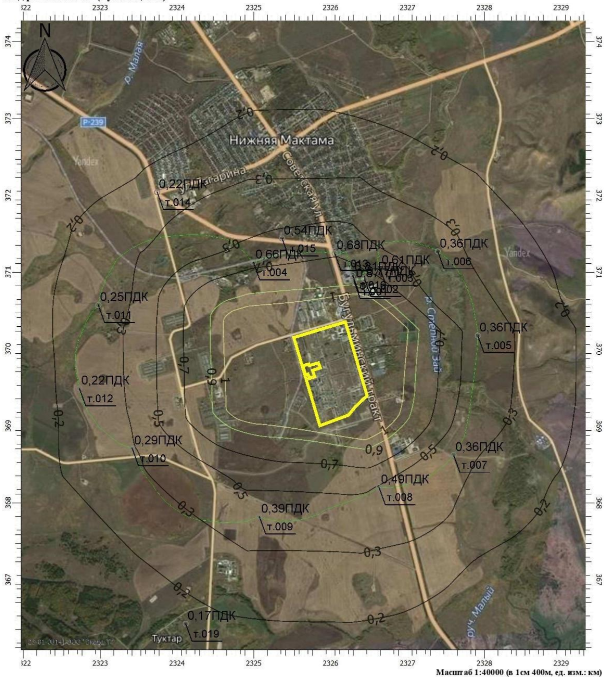
Рисунок 5.1.10 – Карта рассеивания бутилацетата
