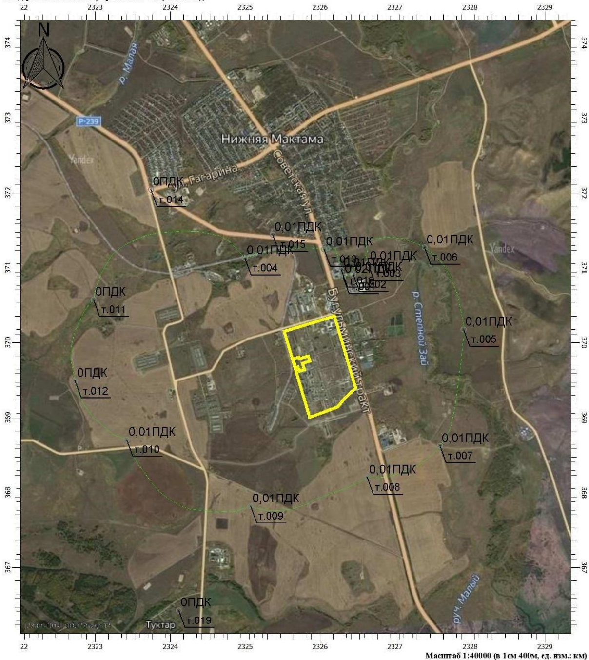
Рисунок 5.1.11 – Карта рассеивания ацетона
