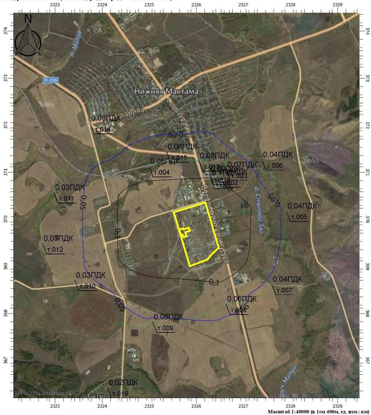
Рисунок 5.1.14 – Карта рассеивания углеводородов предельных C12-C19
