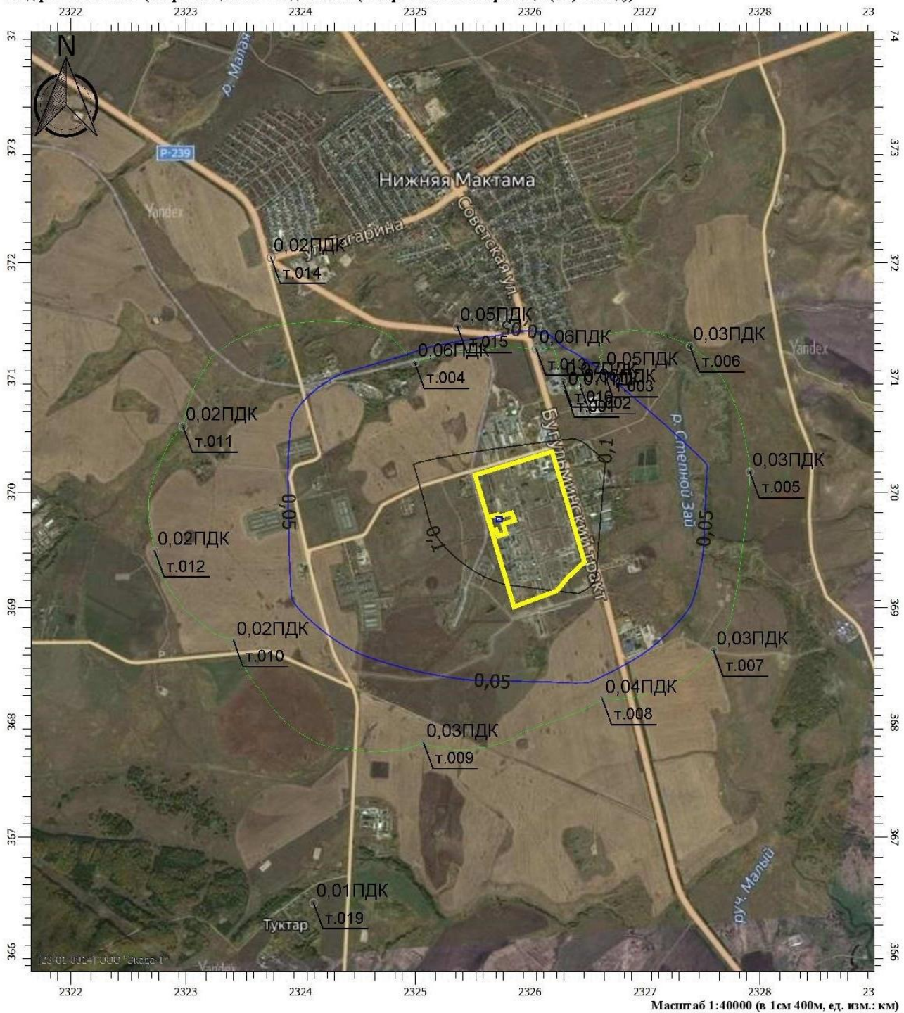
Рисунок 5.1.2 — Карта рассеивания марганца и его соединений
