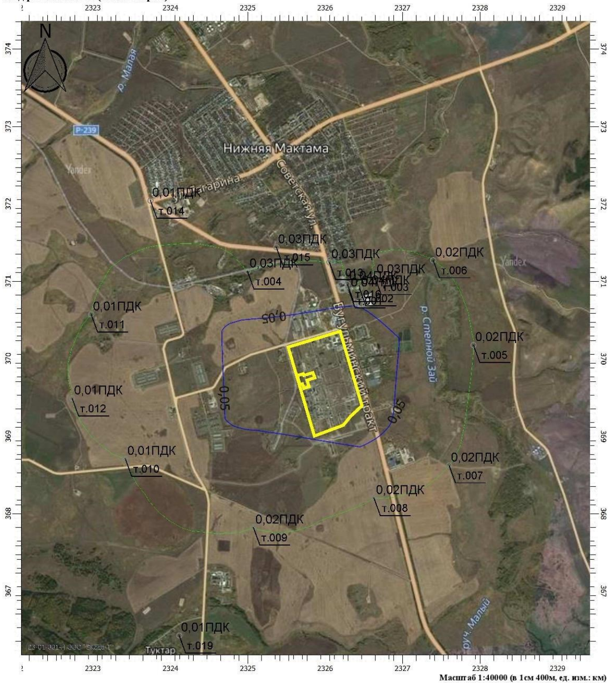
Рисунок 5.1.13 – Карта рассеивания уайт-спирит
