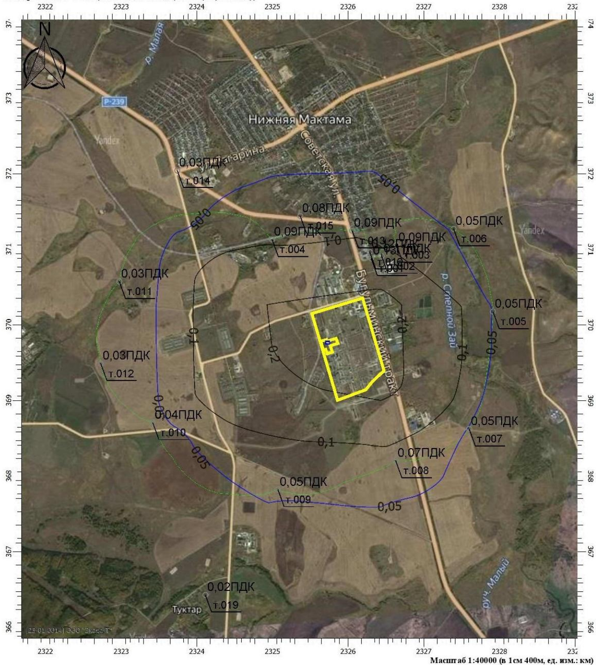
Рисунок 5.1.3 – Карта рассеивания диоксида азота
