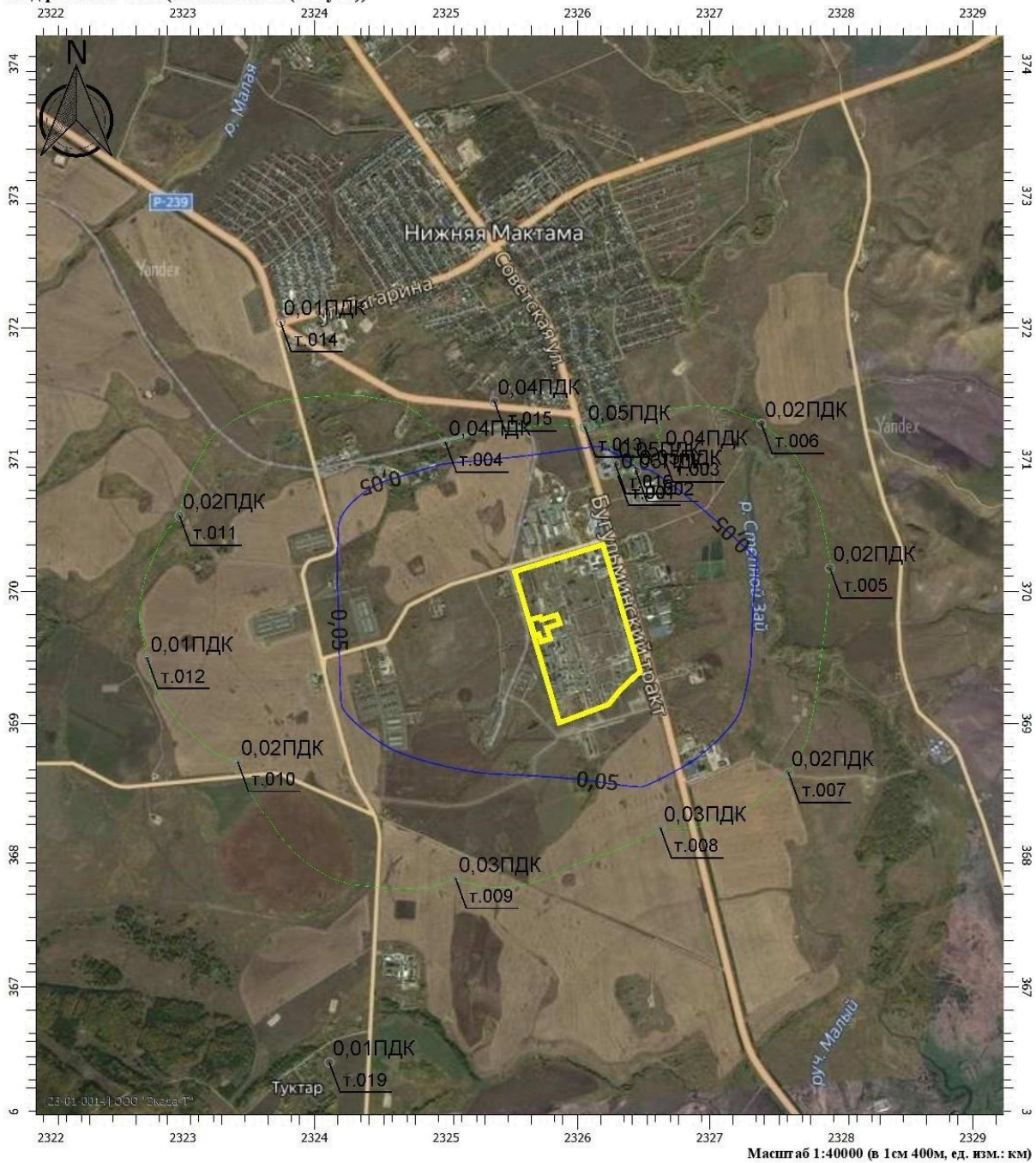
Рисунок 5.1.8 – Карта рассеивания толуола
