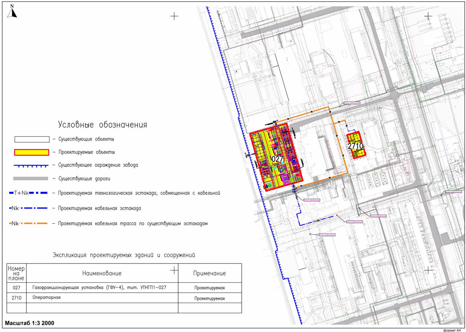
Рисунок 3.2.1 – Генеральный план проектируемой ГФУ-4
