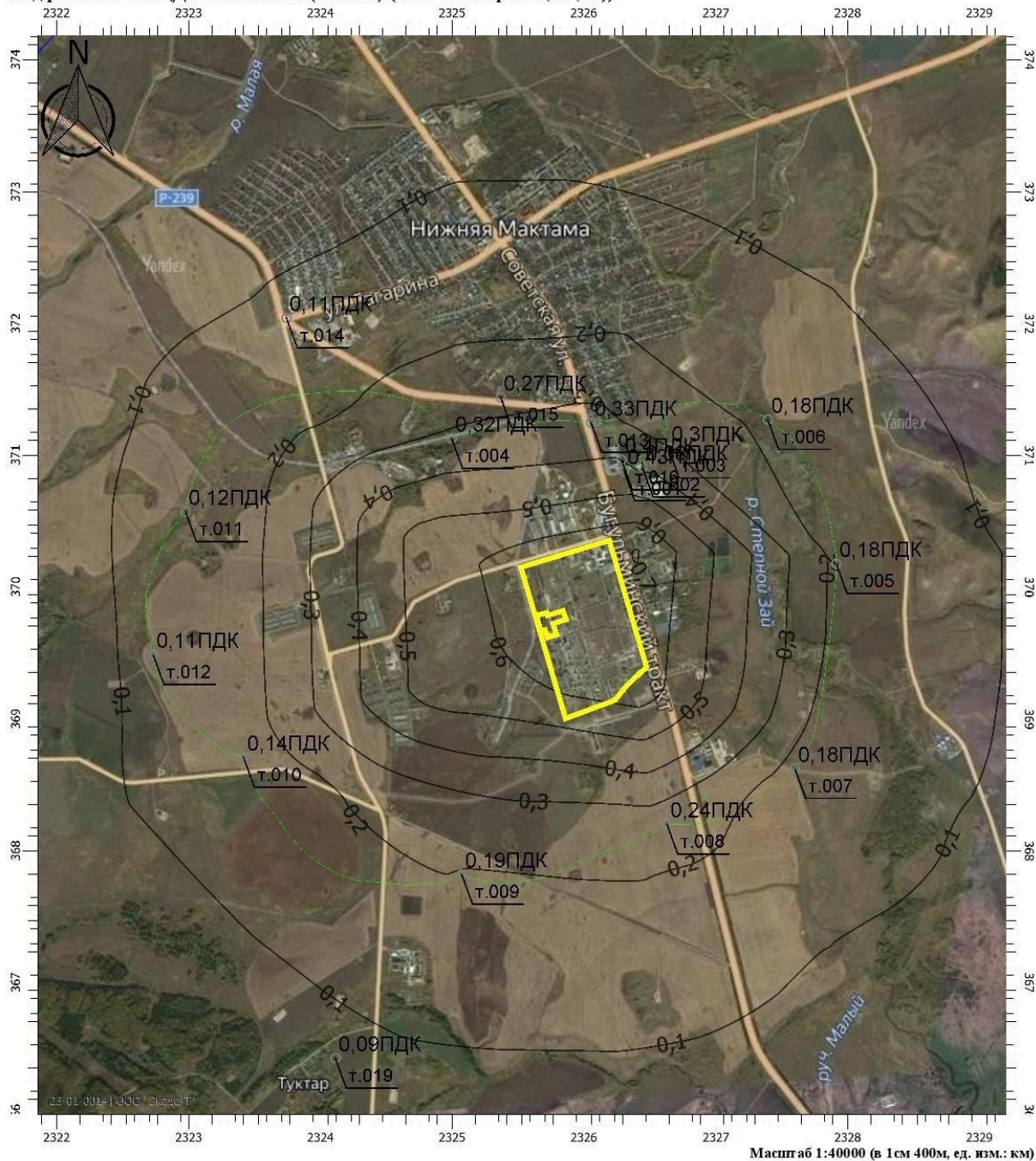
Рисунок 5.1.7 – Карта рассеивания ксилола
